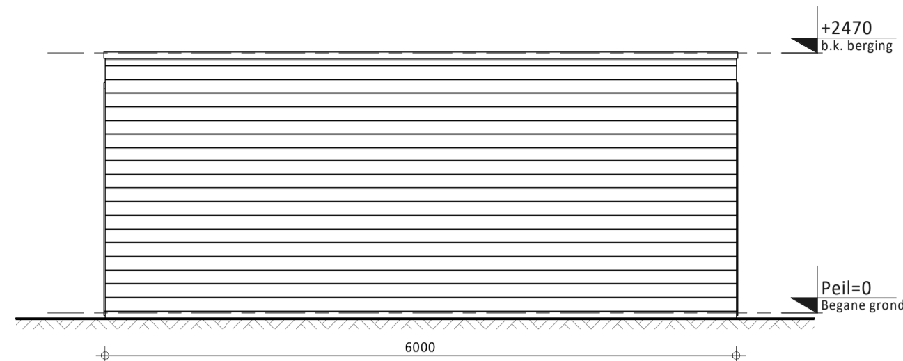
Vooranzicht
