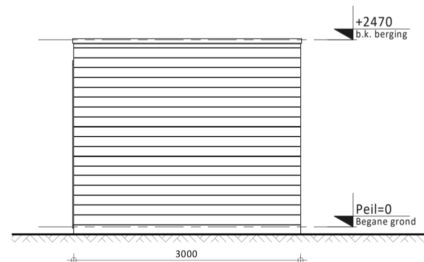
Vooranzicht
