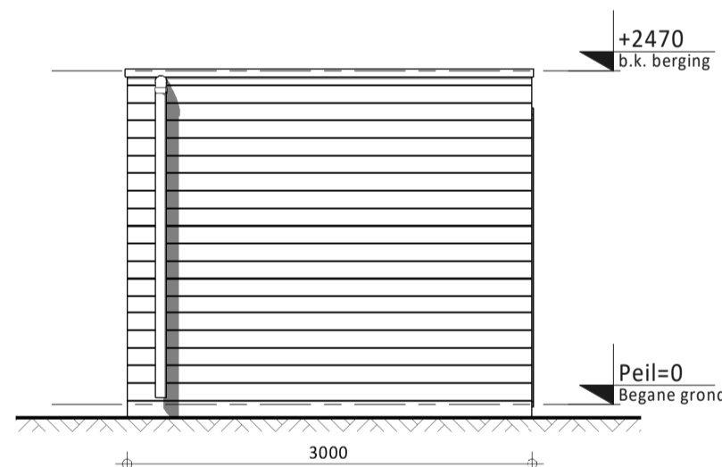
Achteraanzicht
